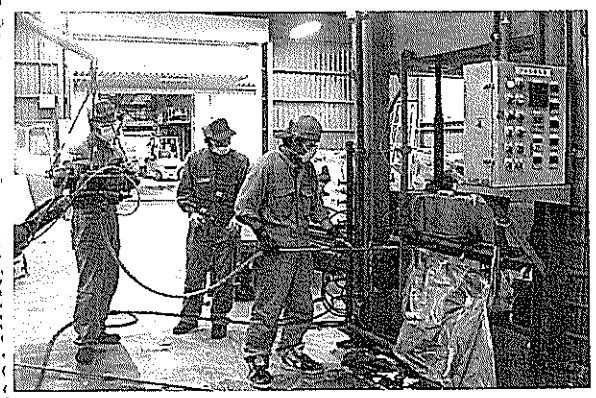
低圧発泡機(左)とプレス機(右)
